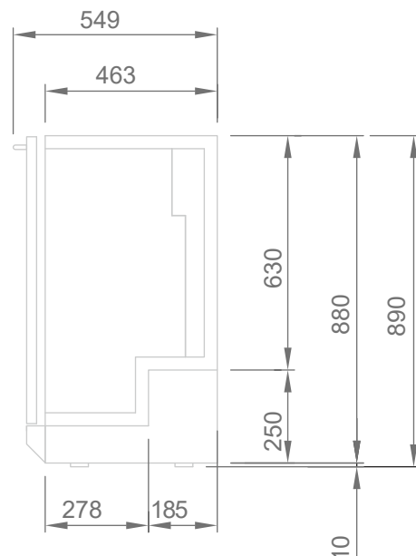
ВИД СБОКУ
