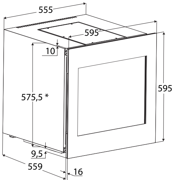
Vista lateral
