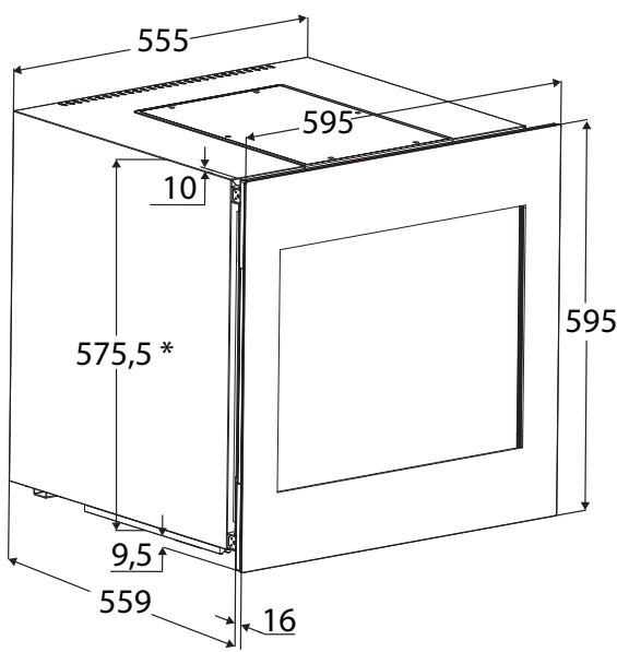
Vista lateral
