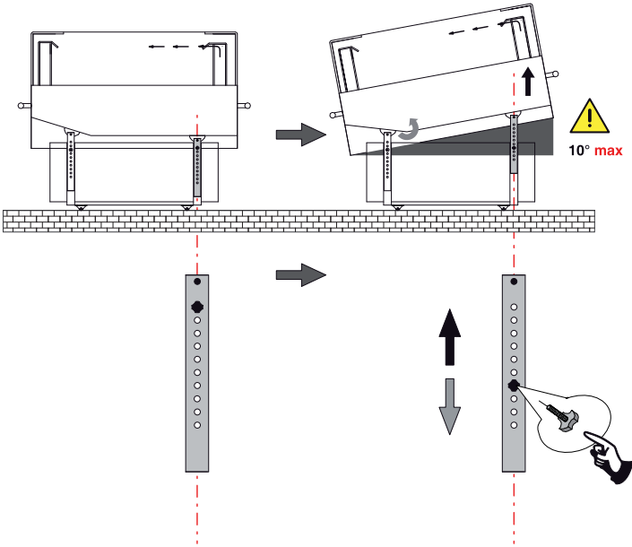
INCLINATION
