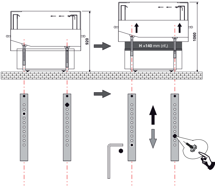
ELEVATION
